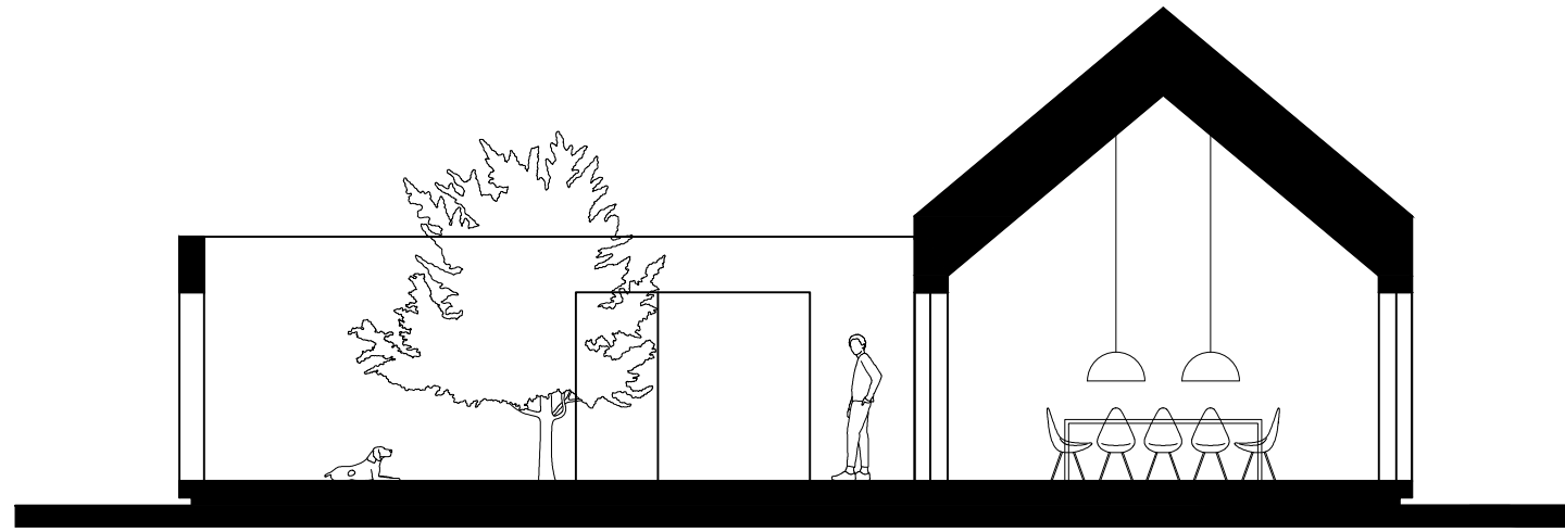
REZ A-A
